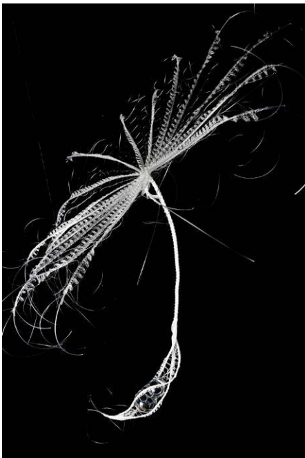
Anémochorie
